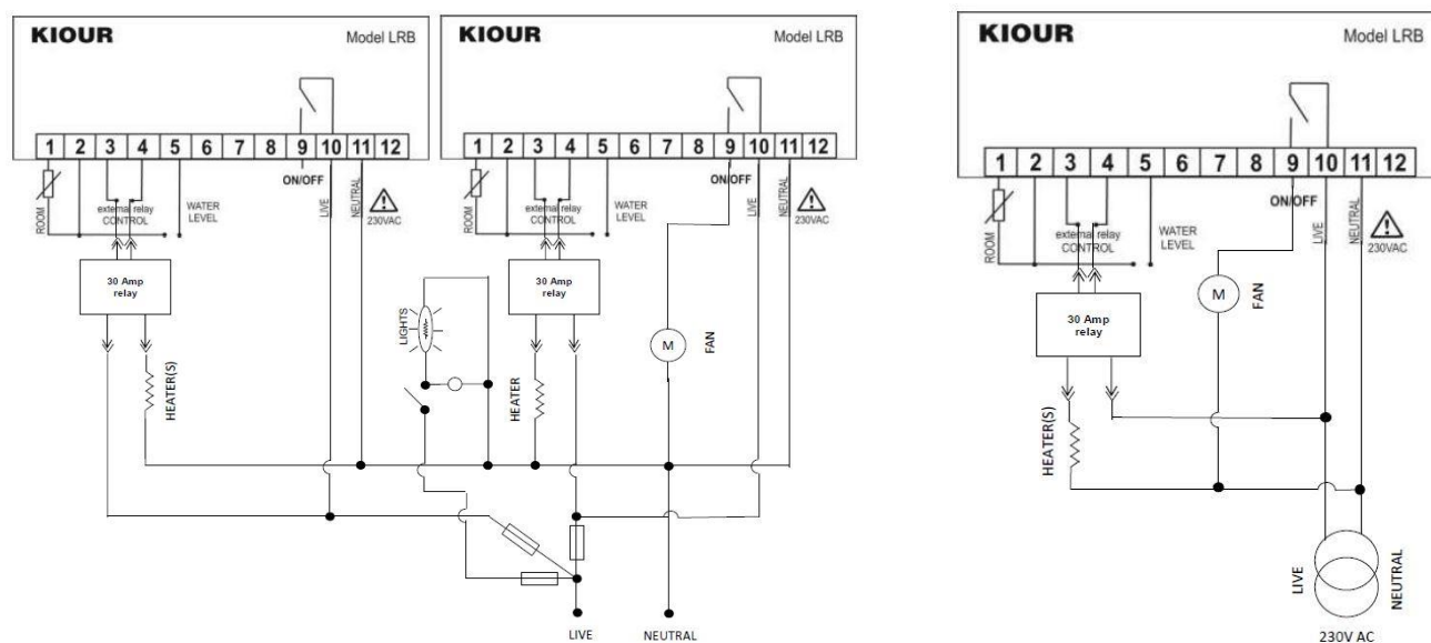
Επιδαπέδια M-M με βιτρίνα με θερμοεγμάριο 1PH
