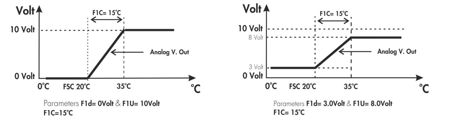
ΣΧΗΜΑ 6Β FAN 1 ΣΤΗΝ ΘΕΡΜΑΝΣΗ ΛΕΙΤΟΥΡΓΙΑ ΚΑΙ ΡΥΘΜΙΣΕΙΣ ΤΗΣ ΑΝΑΛΟΓΙΚΗΣ ΕΞΟΔΟΥ
