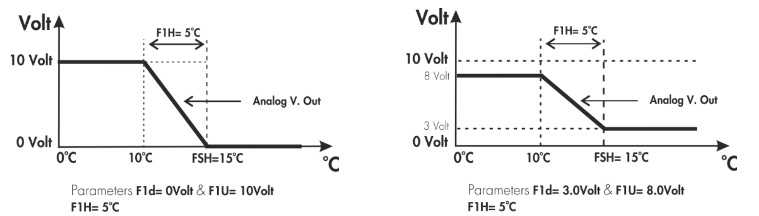
ΣΧΗΜΑ 6Β FAN 1 ΣΤΗΝ ΘΕΡΜΑΝΣΗ ΛΕΙΤΟΥΡΓΙΑ ΚΑΙ ΡΥΘΜΙΣΕΙΣ ΤΗΣ ΑΝΑΛΟΓΙΚΗΣ ΕΞΟΔΟΥ
