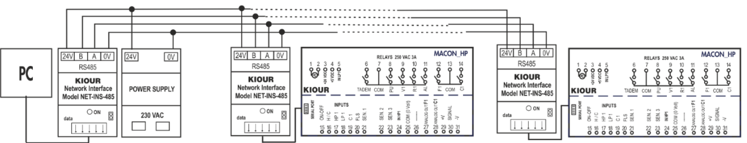
ΣΧΗΜΑ 9 ΣΥΝΔΕΣΜΟΛΟΓΙΑ ΟΡΓΑΝΩΝ ΜΕ ΥΠΟΛΟΓΙΣΤΗ
