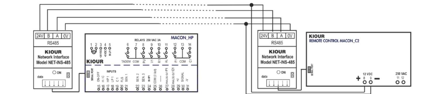
ΣΧΗΜΑ 9 ΣΥΝΔΕΣΜΟΛΟΓΙΑ ΟΡΓΑΝΩΝ ΜΕ ΥΠΟΛΟΓΙΣΤΗ
