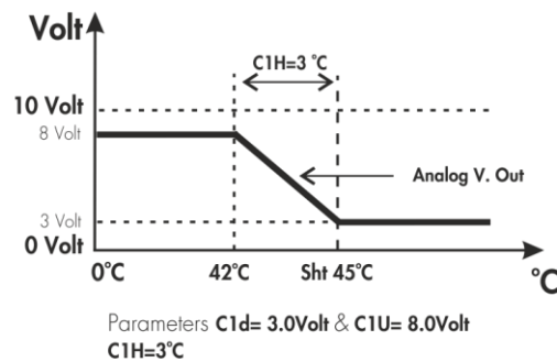
ΣΧΗΜΑ 5Β ΣΥΜΠΙΕΣΤΗΣ C1 ΣΤΗΝ ΘΕΡΜΑΝΣΗ ΛΕΙΤΟΥΡΓΙΑ ΚΑΙ ΡΥΘΜΙΣΕΙΣ ΤΗΣ ΑΝΑΛΟΓΙΚΗΣ ΕΞΟΔΟΥ
