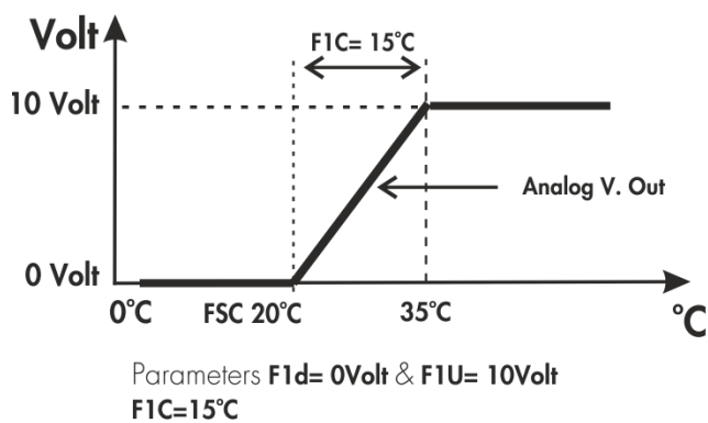
ΣΧΗΜΑ 6Α FAN 1 ΣΤΗΝ ΨΥΞΗ ΛΕΙΤΟΥΡΓΙΑ ΚΑΙ ΡΥΘΜΙΣΕΙΣ ΤΗΣ ΑΝΑΛΟΓΙΚΗΣ ΕΞΟΔΟΥ
