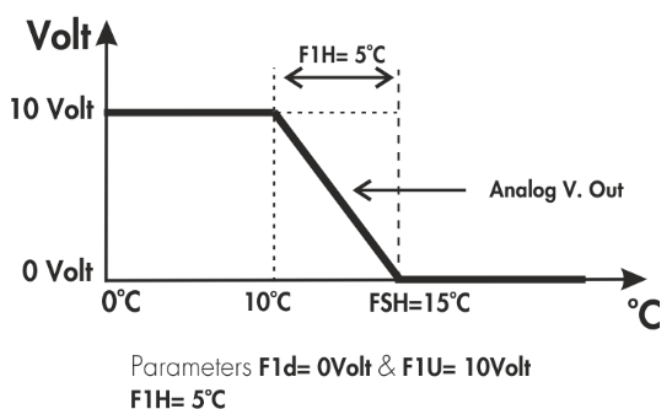
ΣΧΗΜΑ 6Β FAN 1 ΣΤΗΝ ΘΕΡΜΑΝΣΗ ΛΕΙΤΟΥΡΓΙΑ ΚΑΙ ΡΥΘΜΙΣΕΙΣ ΤΗΣ ΑΝΑΛΟΓΙΚΗΣ ΕΞΟΔΟΥ
