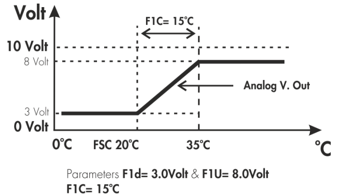
ΣΧΗΜΑ 6Α FAN 1 ΣΤΗΝ ΨΥΞΗ ΛΕΙΤΟΥΡΓΙΑ ΚΑΙ ΡΥΘΜΙΣΕΙΣ ΤΗΣ ΑΝΑΛΟΓΙΚΗΣ ΕΞΟΔΟΥ
