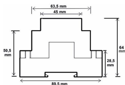
ΣΧΗΜΑ 3 ΔΙΑΣΤΑΣΕΙΣ
