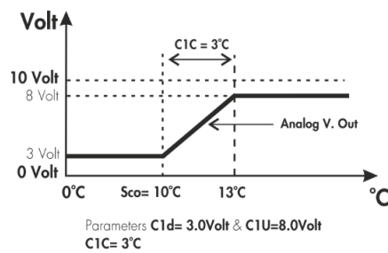
ΣΧΗΜΑ 5Α ΣΥΜΠΙΕΣΤΗΣ C1 ΣΤΗΝ ΨΥΞΗ ΛΕΙΤΟΥΡΓΙΑ ΚΑΙ ΡΥΘΜΙΣΕΙΣ ΤΗΣ ΑΝΑΛΟΓΙΚΗΣ ΕΞΟΔΟΥ
