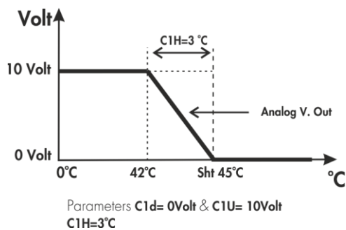
ΣΧΗΜΑ 5Β ΣΥΜΠΙΕΣΤΗΣ C1 ΣΤΗΝ ΘΕΡΜΑΝΣΗ ΛΕΙΤΟΥΡΓΙΑ ΚΑΙ ΡΥΘΜΙΣΕΙΣ ΤΗΣ ΑΝΑΛΟΓΙΚΗΣ ΕΞΟΔΟΥ
